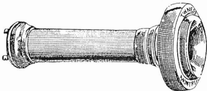
STANDARD H. M. B. RECEIVER
